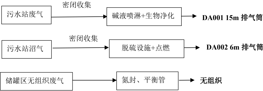
图 8-1 本项目废气收集及治理走向示意图
