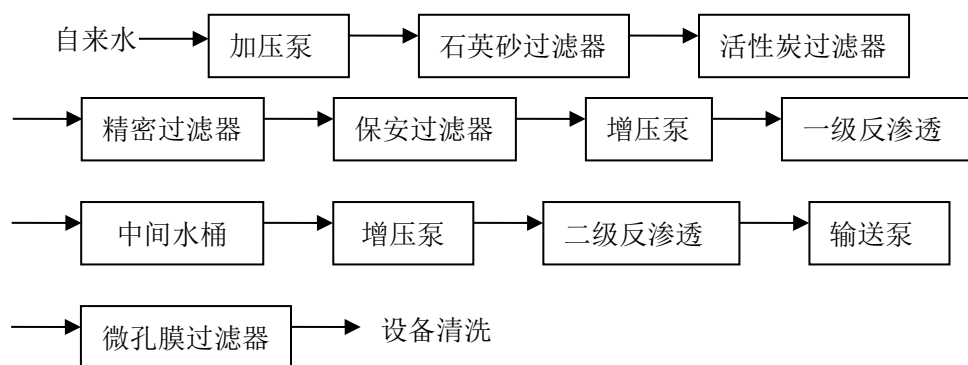
图 4.2-1 纯化水工艺流程示意图
