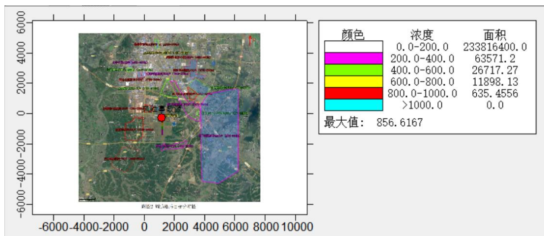
图 9-2 储罐区甲醇泄漏等值线分布图（最不利气象）
