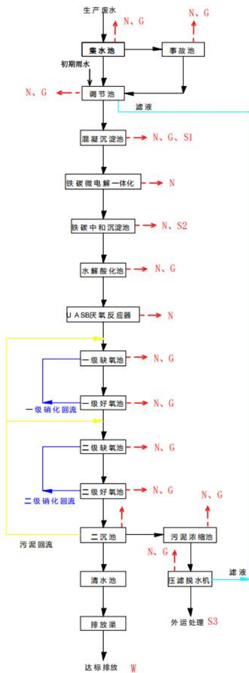
图 4.1-1 污水处理工艺流程及产污节点图
