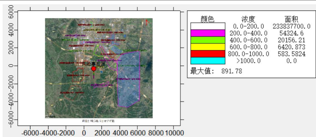
图 9-1 储罐区氨水泄漏等值线分布图（最不利气象）
